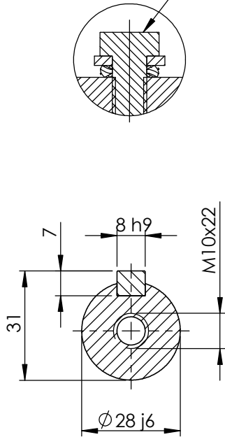
SECTION A-A SCALE 1 : 1.5
