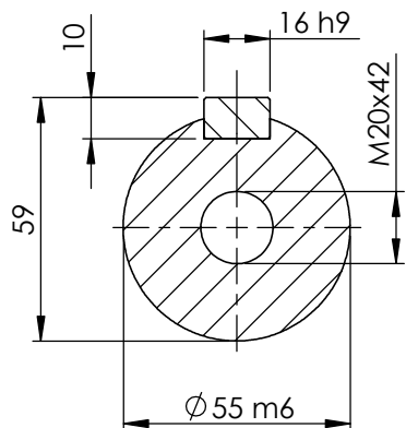
SECTION A-A SCALE 1 : 2
