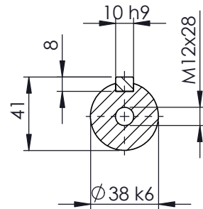
SECTION A-A SCALE 1 : 3
