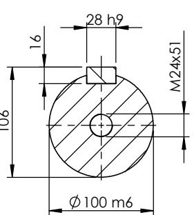
SECTION A-A SCALA 1 : 5
