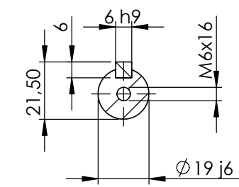
SEZIONE A-A SCALA 1 : 2
