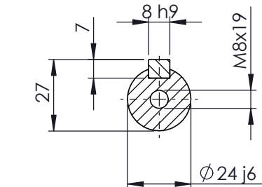
SECTION A-A SCALE 1 : 2
