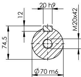
SEZIONE A-A SCALA 1 : 5
