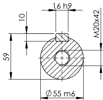
SECTION A-A SCALE 1 : 3
