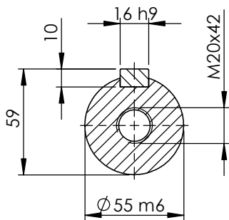
SECTION A-A SCALE 1 : 3
