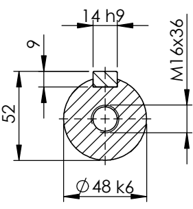
SECTION A-A SCALE 1 : 3
