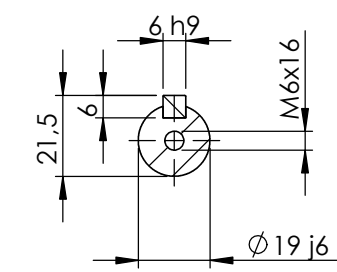
SEZIONE A-A SCALA 1 : 2
