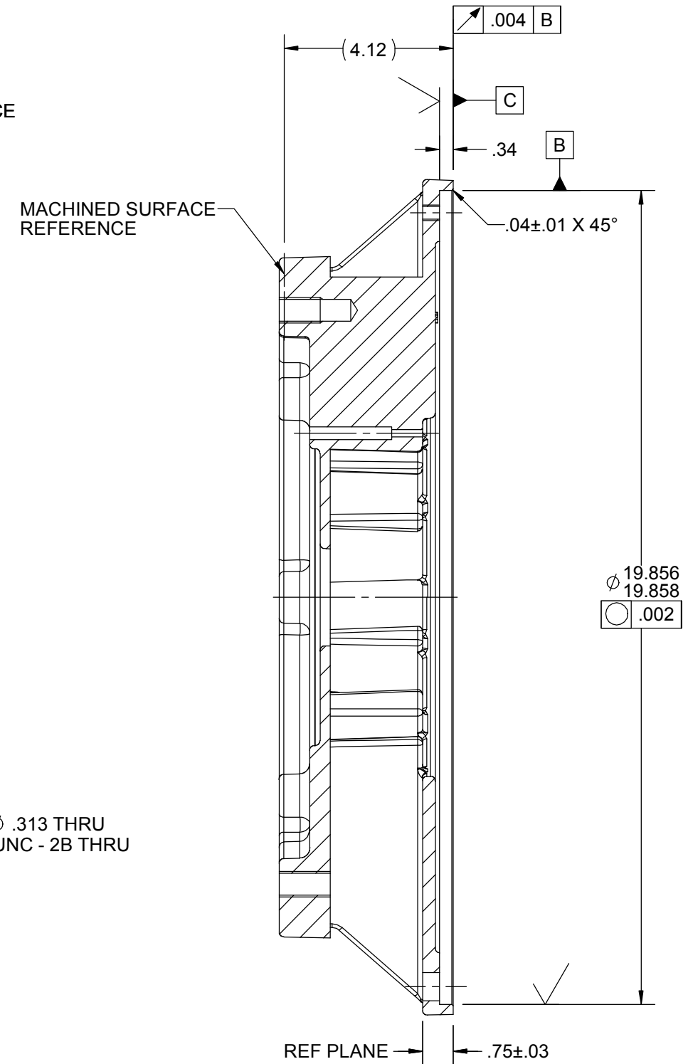
SECTION A-A
