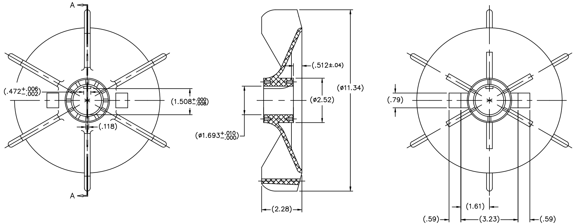
SECTION A-A
