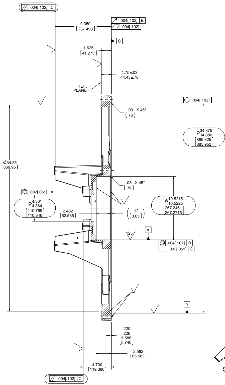
SECTION A-A
